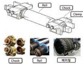
제철설비(롤설비)
