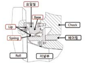
제철설비(철구조)
